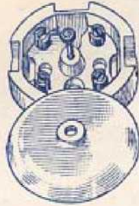
N° 301 BOITE RONDE avec entrées de tube couvercle porcelaine le cent ..... 100. » N° 333 — — — — — tôle ..... 135. »
