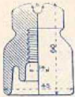
N° 305 DOUBLE CLOCHE 45×60, le cent 60. » N° 306 60×80, — 95. » N° 307 70×100, — 135. » N° 308 125×70, — 280. » N° 309 130×80, — 365. »
